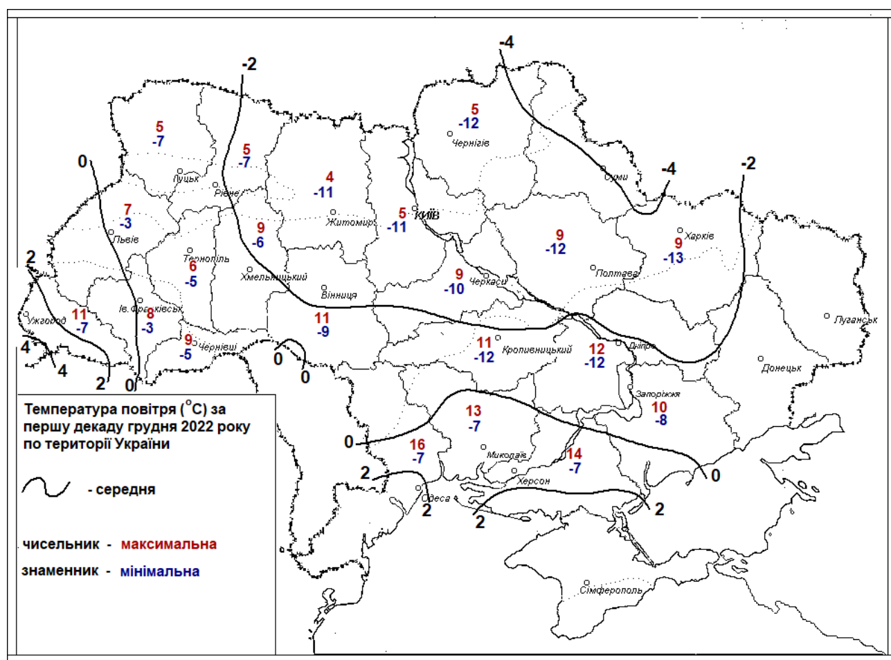
Рис.1 Температура повітря (°С) за першу декаду грудня 2022 року по території України
