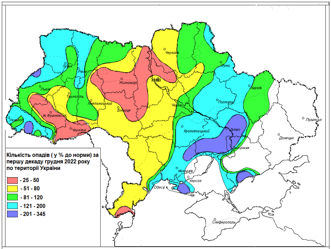
Рис.2 Кількість опадів (% до норми) за першу декаду грудня 2022 року по території України
