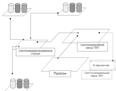
Рис.2. Концептуальна модель організації системи переробки ТПВ на регіональному рівні
